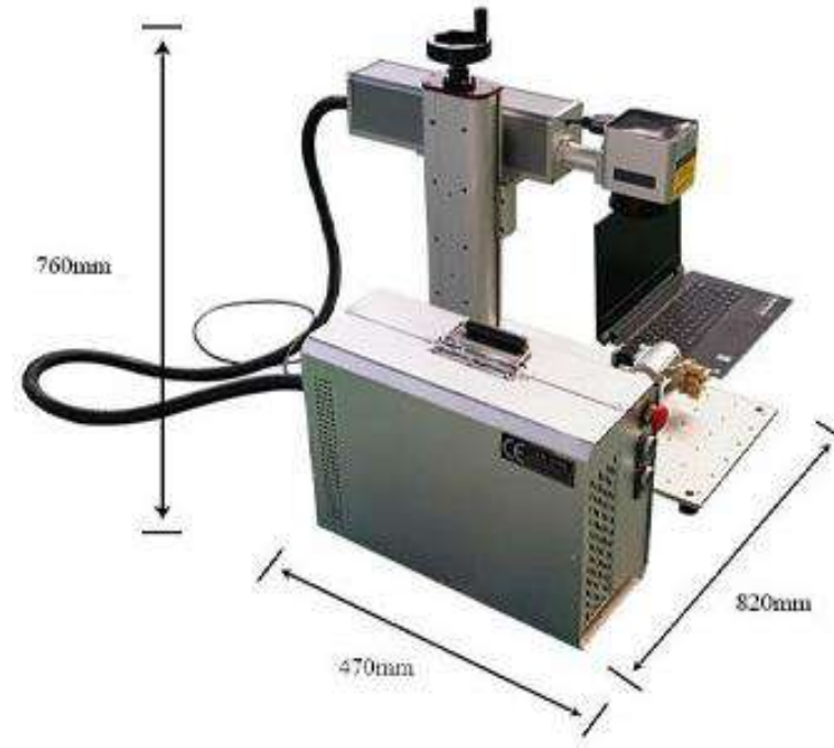
Portable Mini Desktop Fiber Laser Marking
